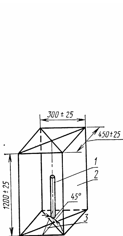
1—образец кабеля; 2—испытательная камера; 3—ось горелки Черт. 1
