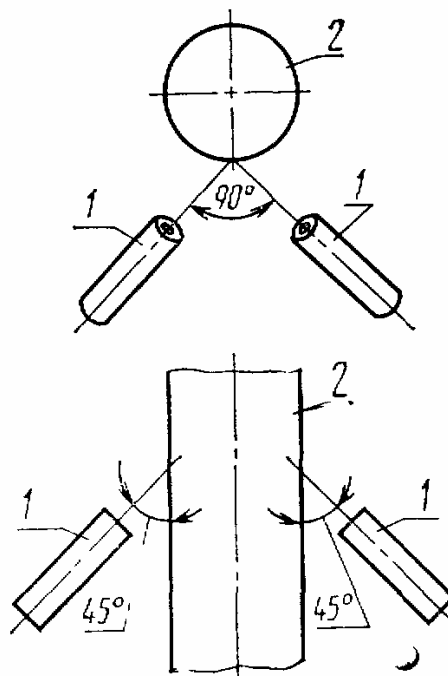
1—горелка; 2—образец Черт. 3
