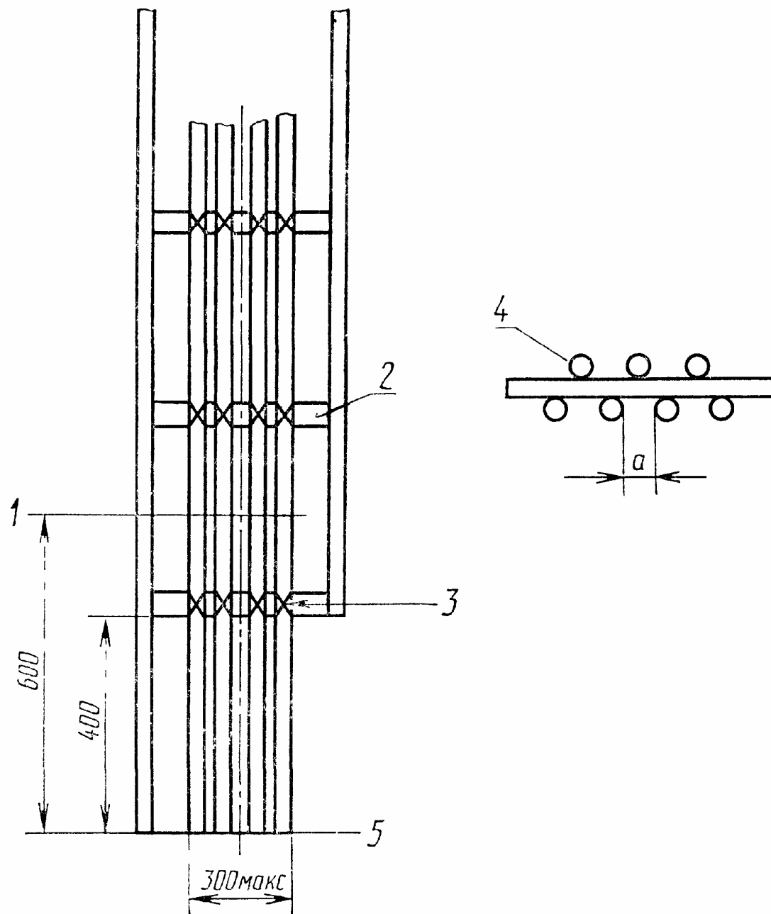
1—центральная линия горелки; 2—круглые стальные перекладки; 3— стальные проволочные крепления; 4— способ расположения кабелей на обеих сторонах лестницы; 5—пол; а—расстояние между закрепленными образцами Черт. 5
