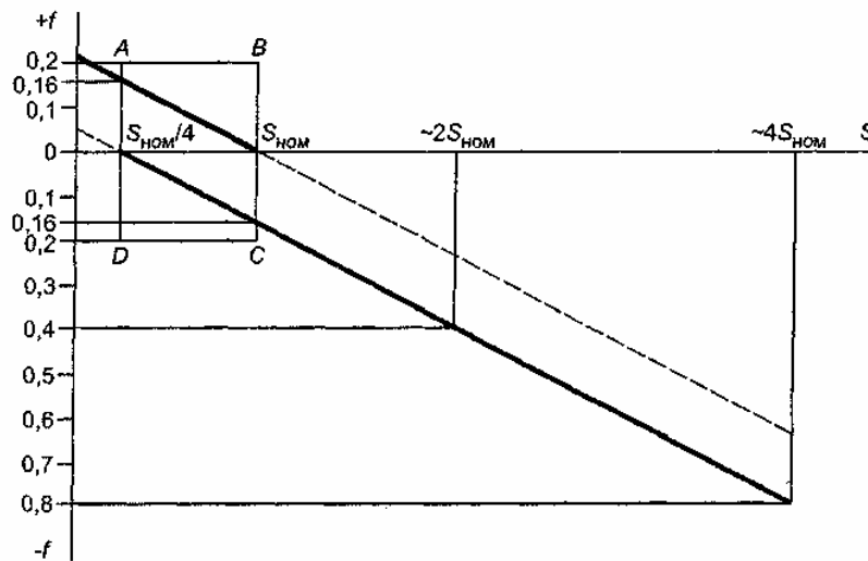
f — погрешность напряжения, %; S_{\text{НОМ}} — номинальная мощность для высшего класса точности, В·А
